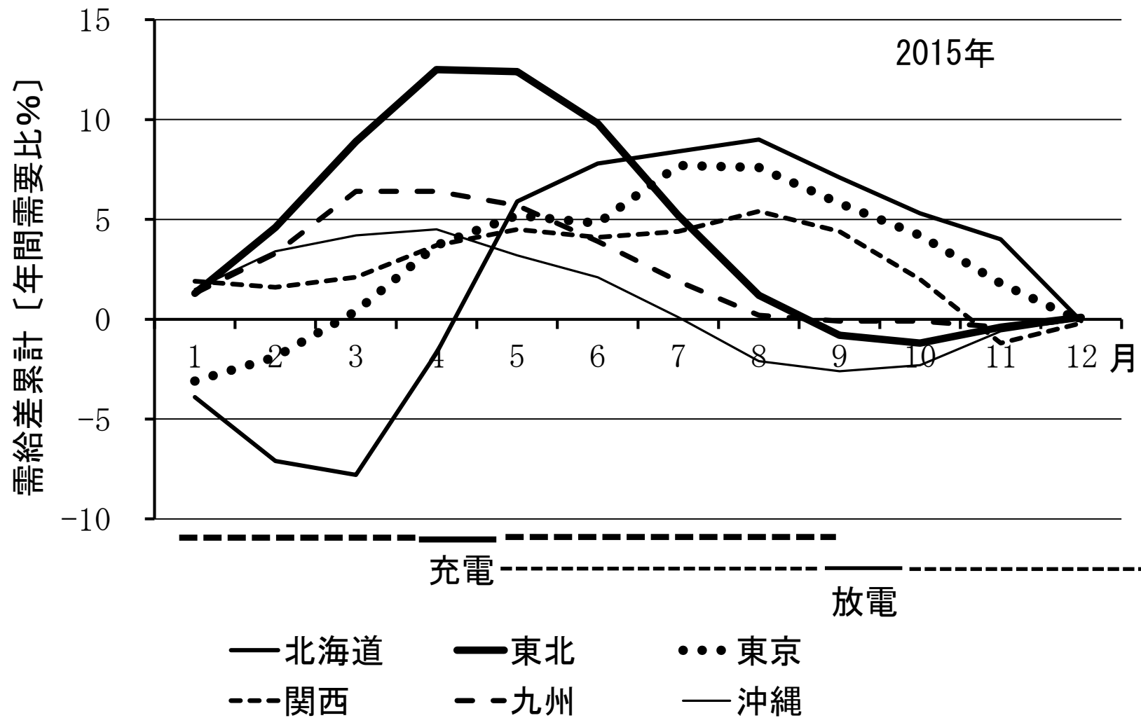
図18 各地域風力発電需給差累計
