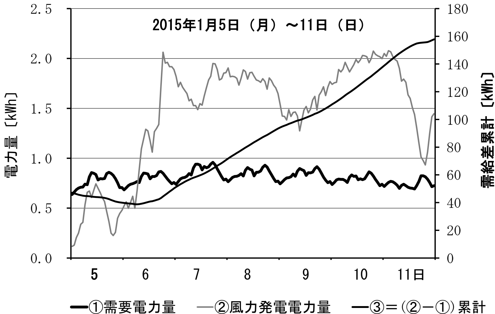
図12 風力発電供給モデル (2)
